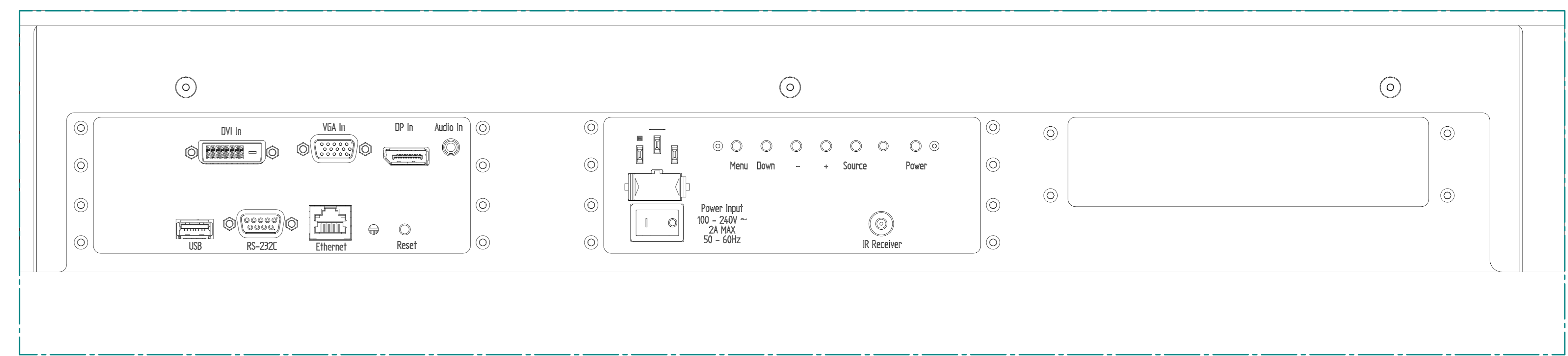
DETAIL A 1:1
