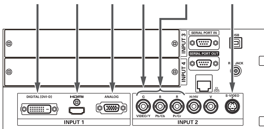
Anschlussbuchsen des Projektors
